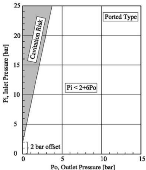
شکل ۸: منحنی کاویتاسیون شیرهای فشار شکن
