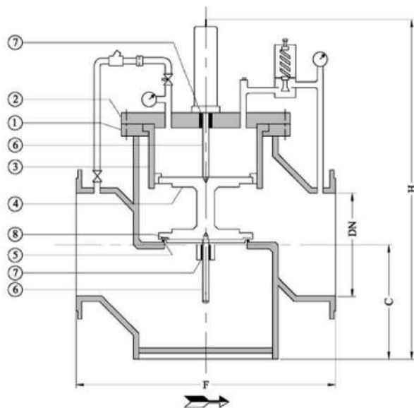
شکل ۱: شیر فشار شکن فولادی پیلوت دار
