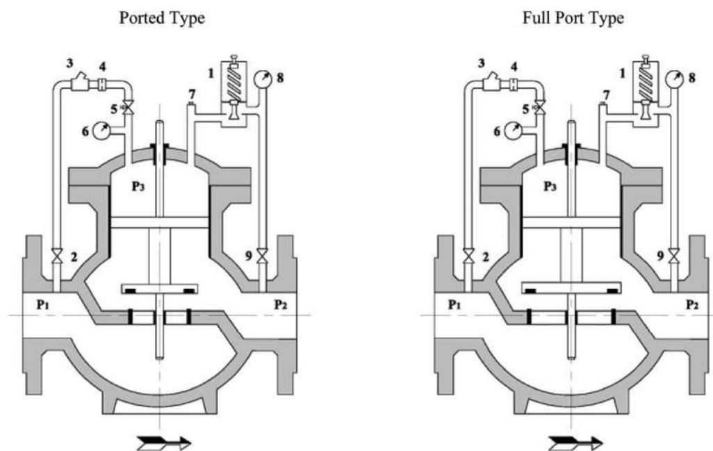
شکل ۳: شیر فشار شکن پیلوت دار*
